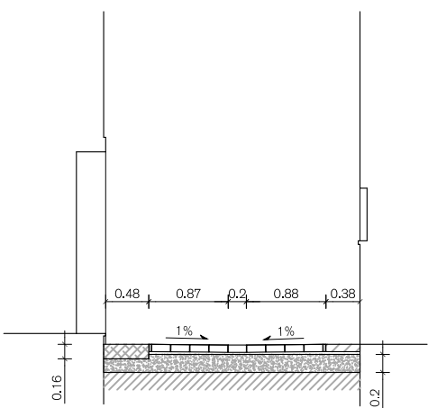
Carrer Dominics, Secció 2 (1:75)
