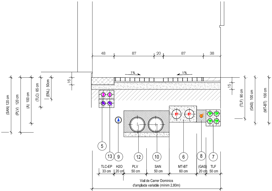
Carrer Dominics, Secció 1 (1:40)
