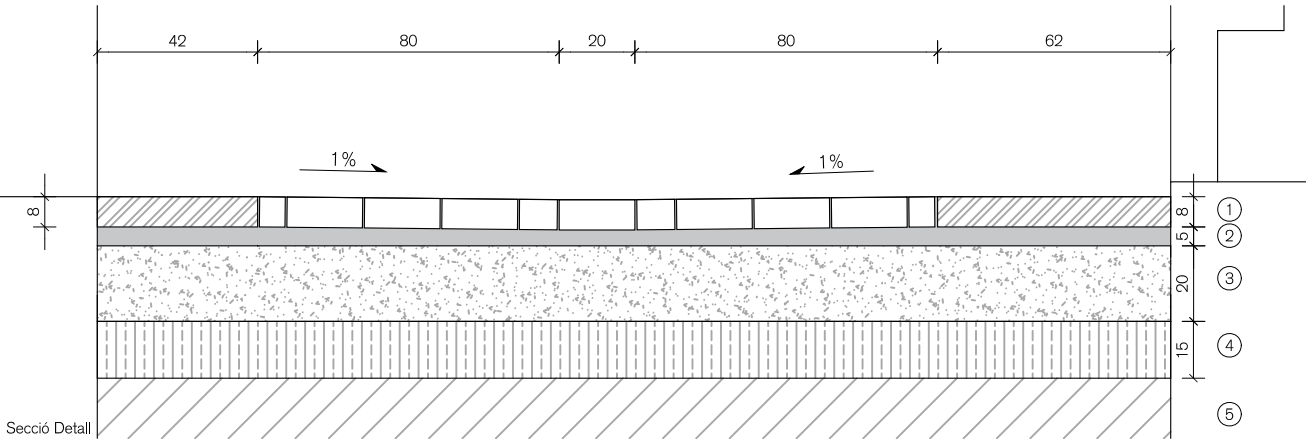
Secció Detall
