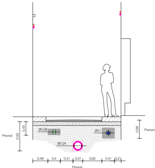
Carrer Dominics, Secció 1 (1:75)
