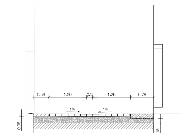
Carrer Dominics, Secció 4 (1:75)
