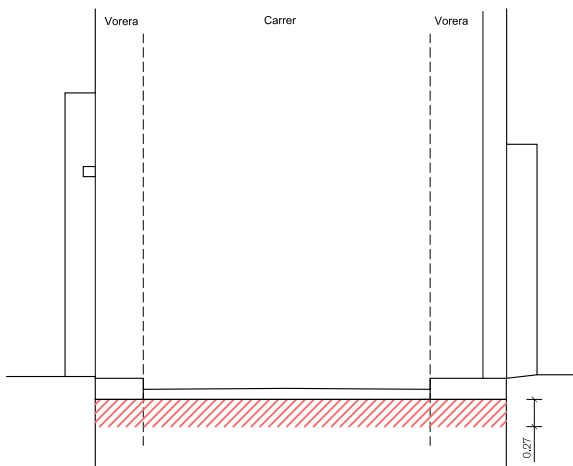
Carrer Dominics, Secció 3 (1:75)
