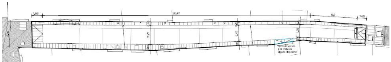
Carrer dels Dominics, planta
