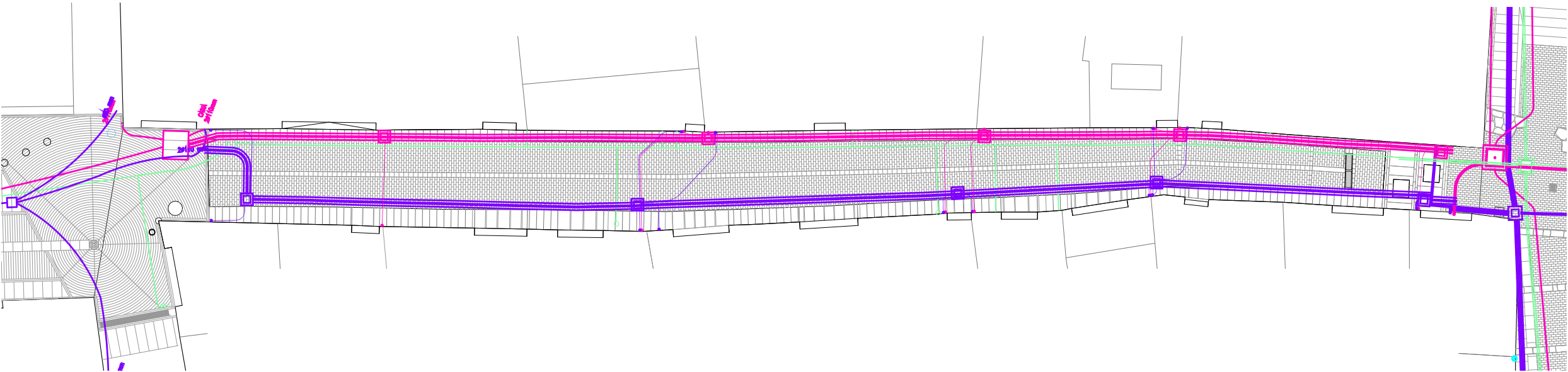
Planta Instal·lacions, Gas, TV, i Telefònica (1:200)
