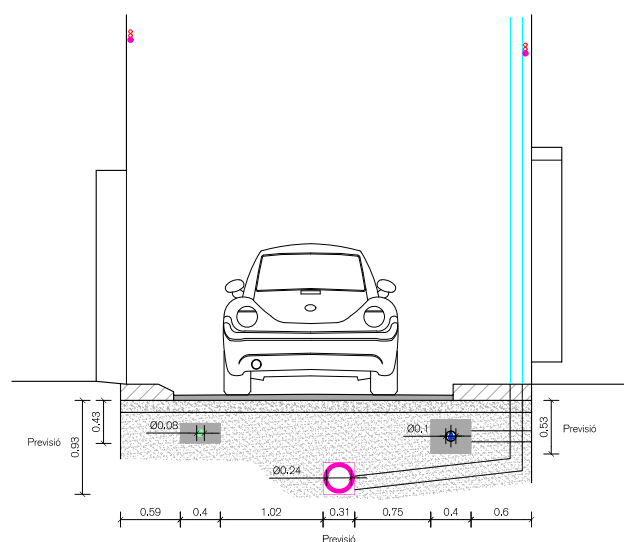
Carrer Dominics, Secció 4 (1:75)
