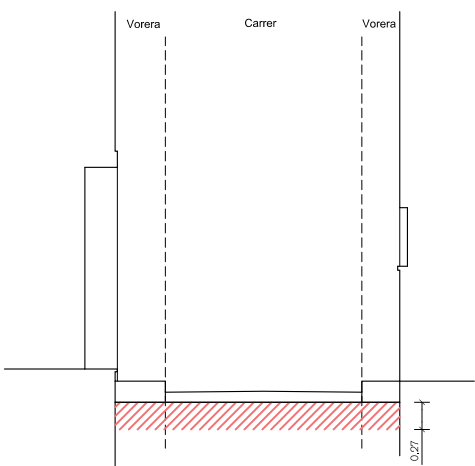
Carrer Dominics, Secció 2 (1:75)
