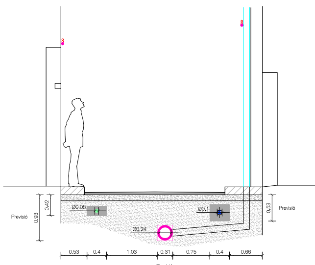
Carrer Dominics, Secció 3 (1:75)
