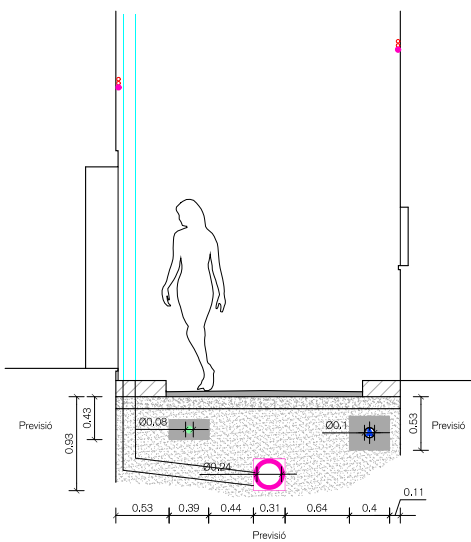
Carrer Dominics, Secció 2 (1:75)
