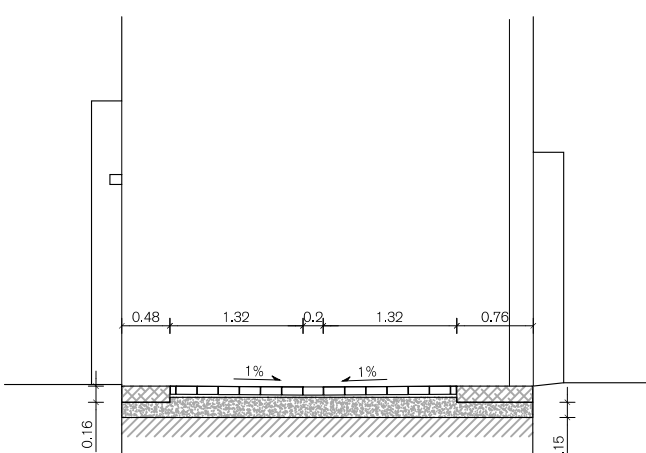
Carrer Dominics, Secció 3 (1:75)
