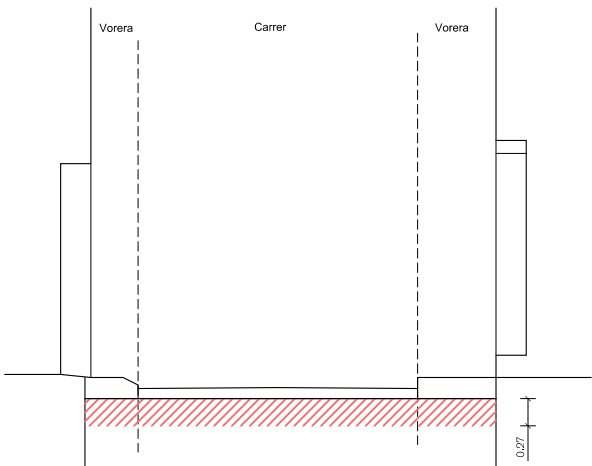
Carrer Dominics, Secció 4 (1:75)
