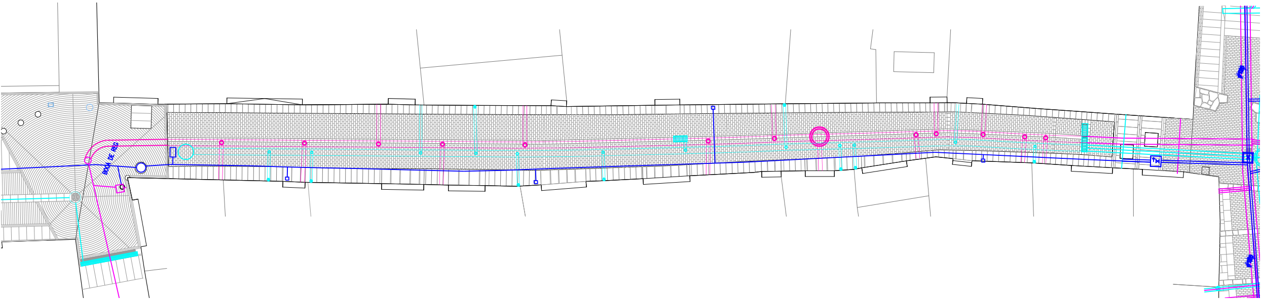
Planta Instal·lacions, aigües negres, pluvials i potable (1:200)
