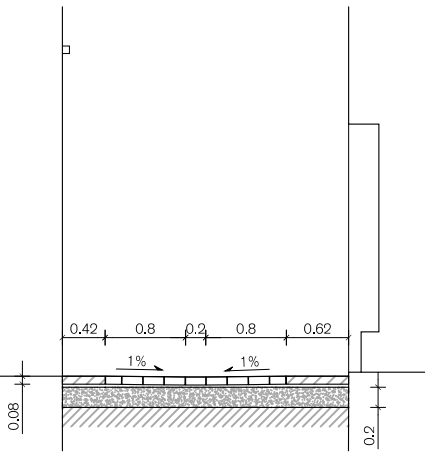
Carrer Dominics, Secció 1 (1:75)
